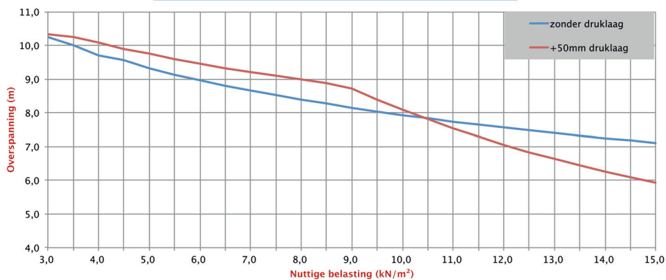
Overspanningsmogelijkheden FS200-600
