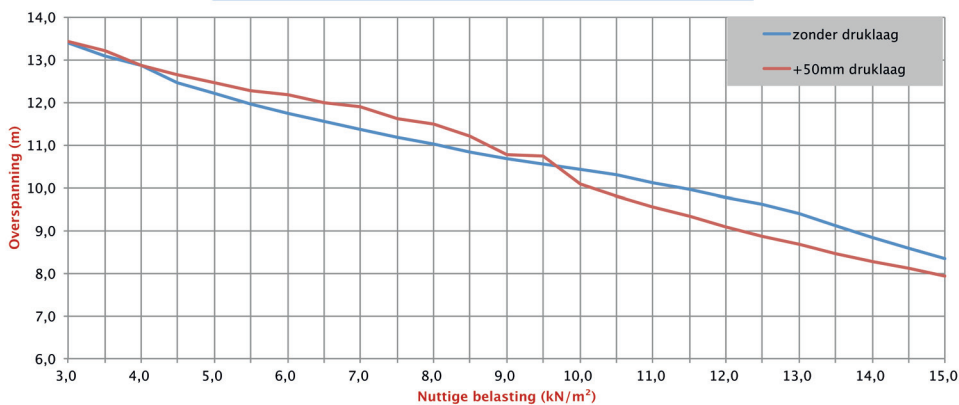
Overspanningsmogelijkheden FS265-1200
