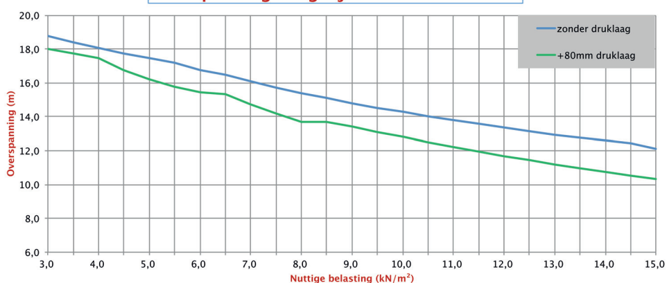
Overspanningsmogelijkheden FS400-1200
